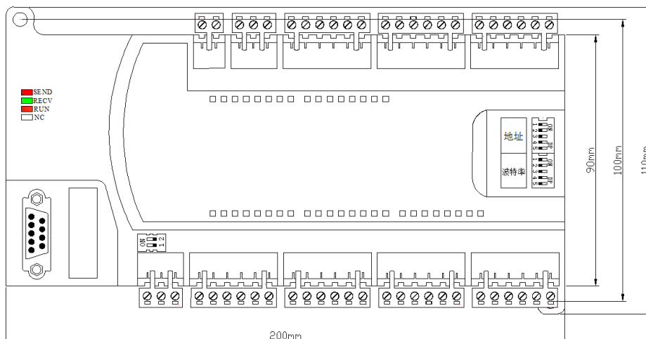
模块尺寸示意图
