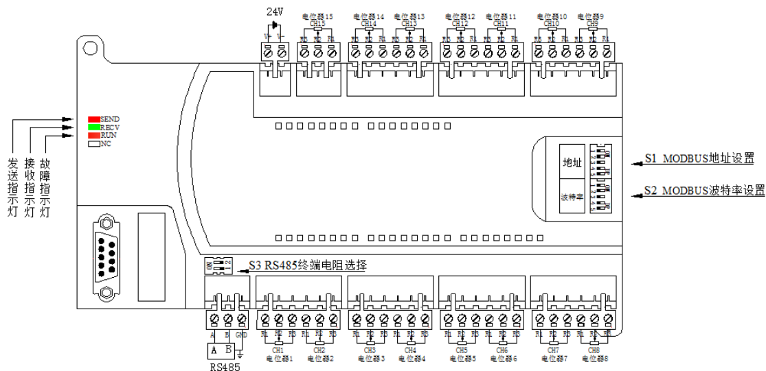
模块接线示意图
